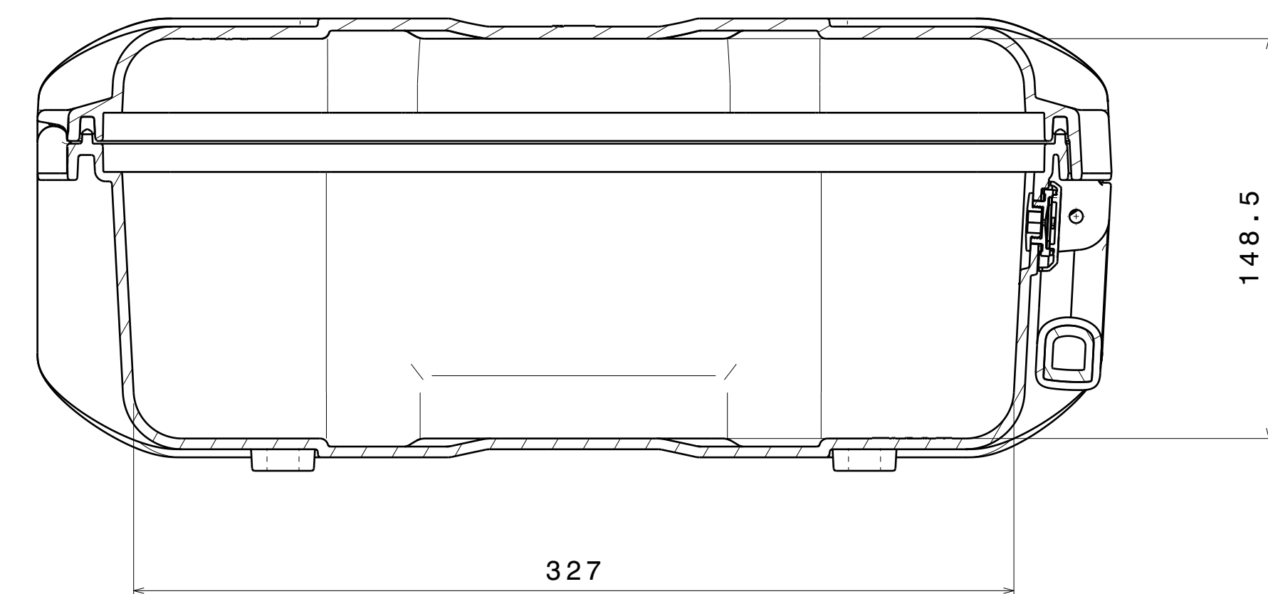
Schnittansicht A-A
