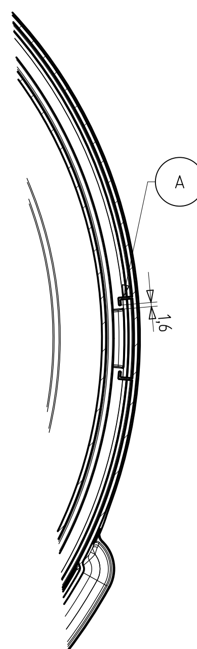
Schnitt AB-AB
