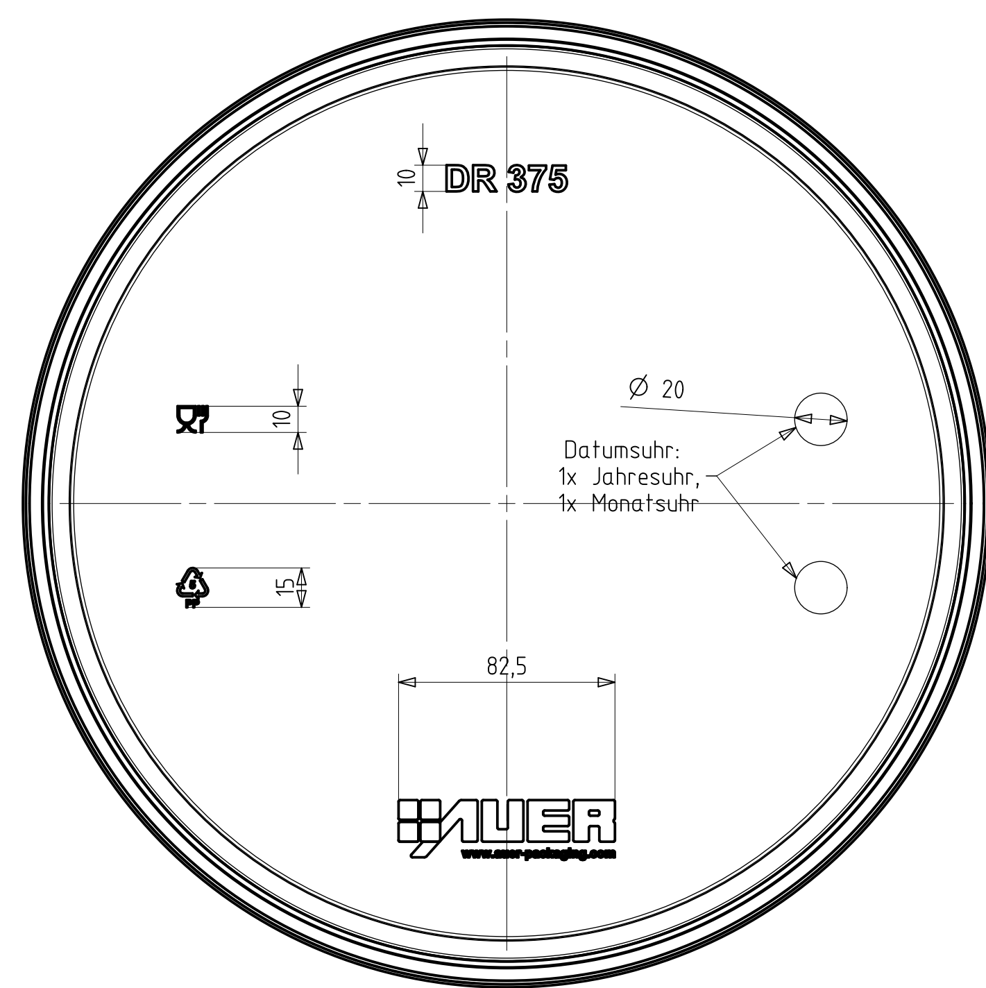
Ansicht Deckel von unten
