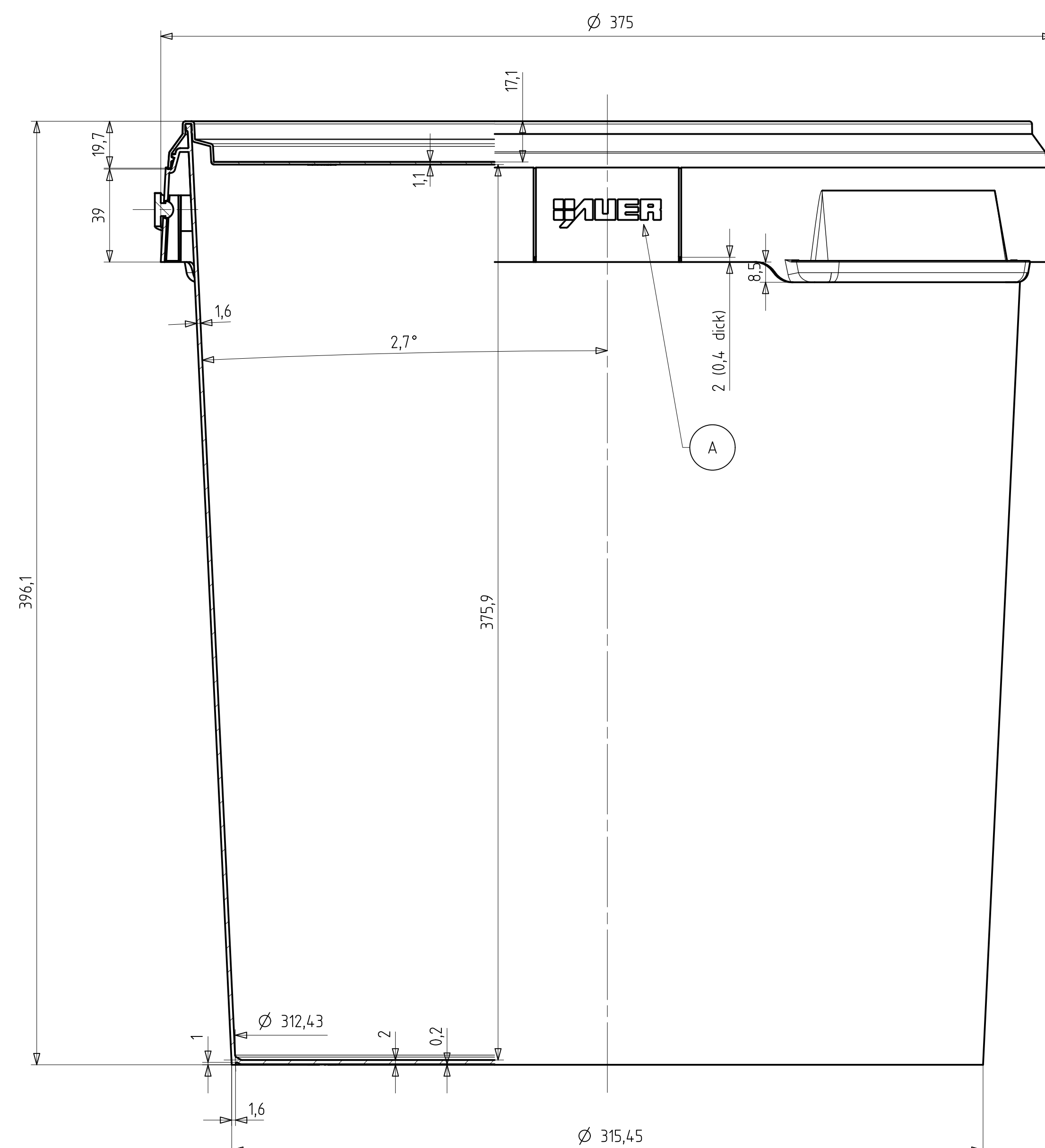
Schnitt A-A
