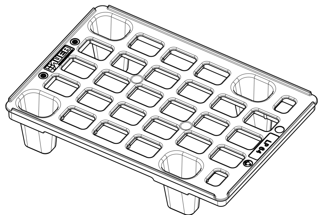
Leichtpalette LP64 mit Sicherungsrand Isometrische Ansicht Maßstab: 1:5
