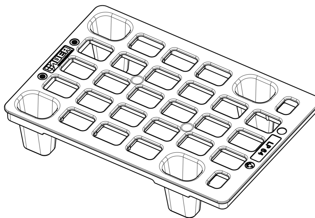
Leichtpalette LP64 OS ohne Sicherungsrand Isometrische Ansicht Maßstab: 1:5
