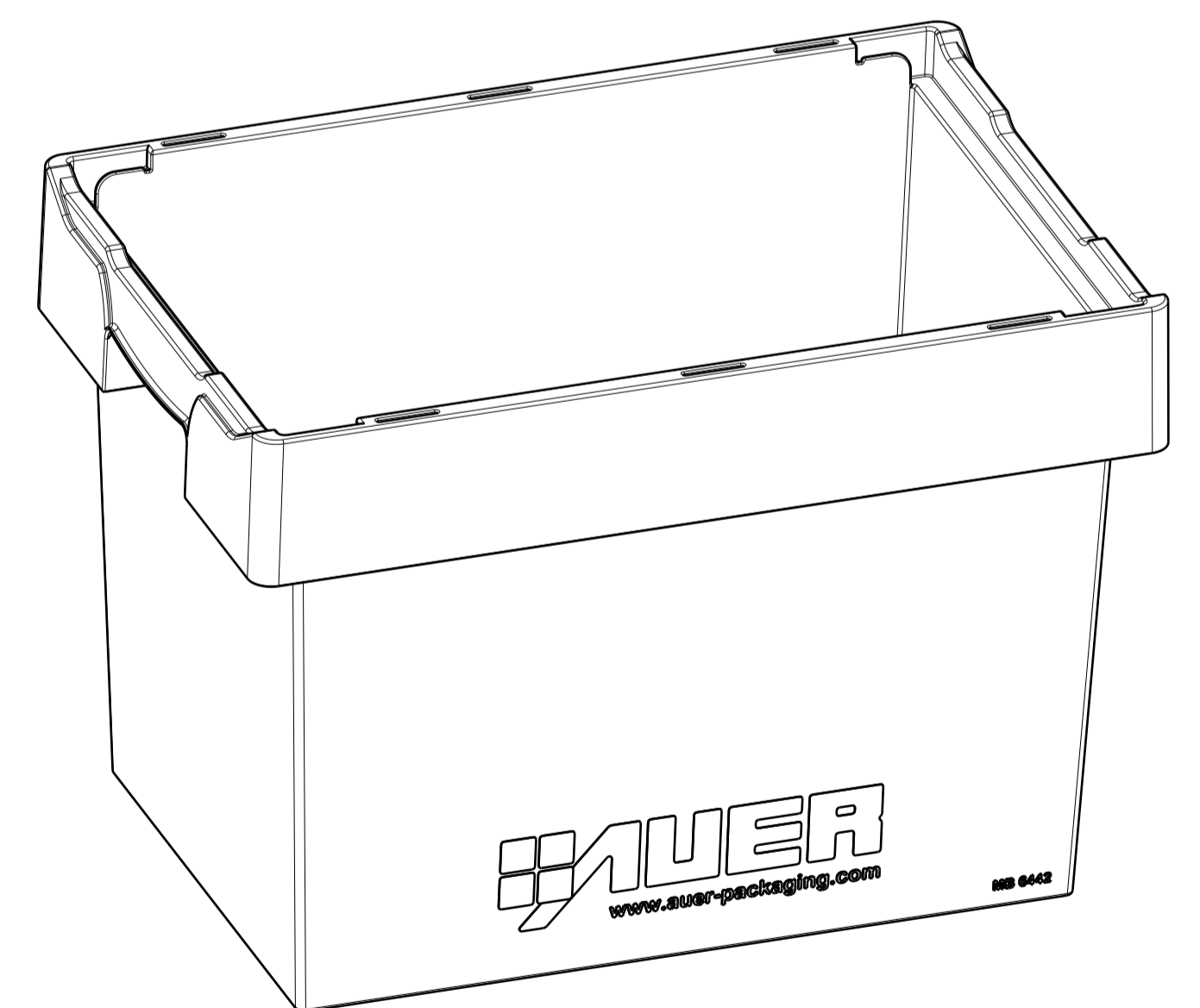
Isometrische Ansicht Maßstab: 1:4
