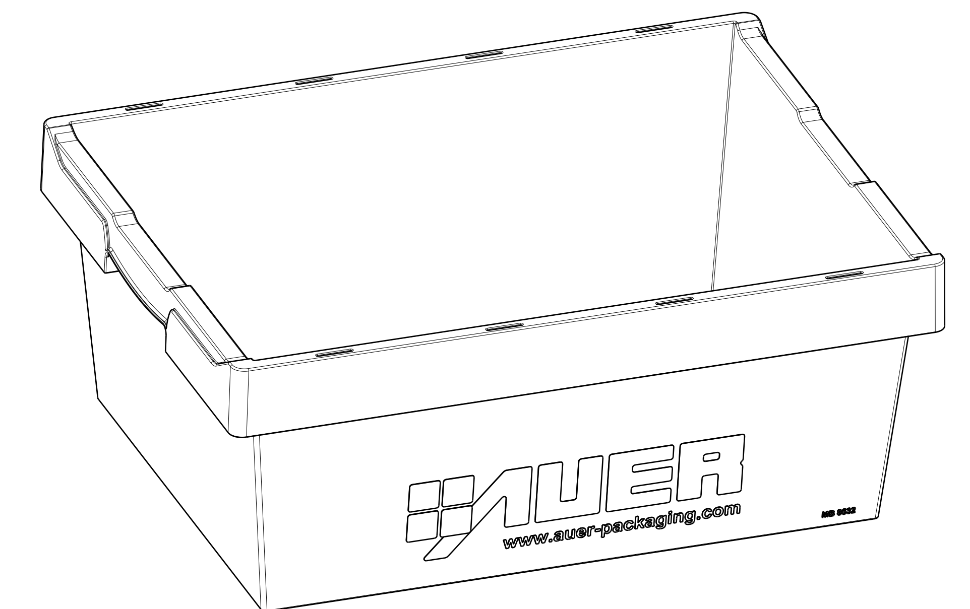
Isometrische Ansicht Maßstab: 1:4
