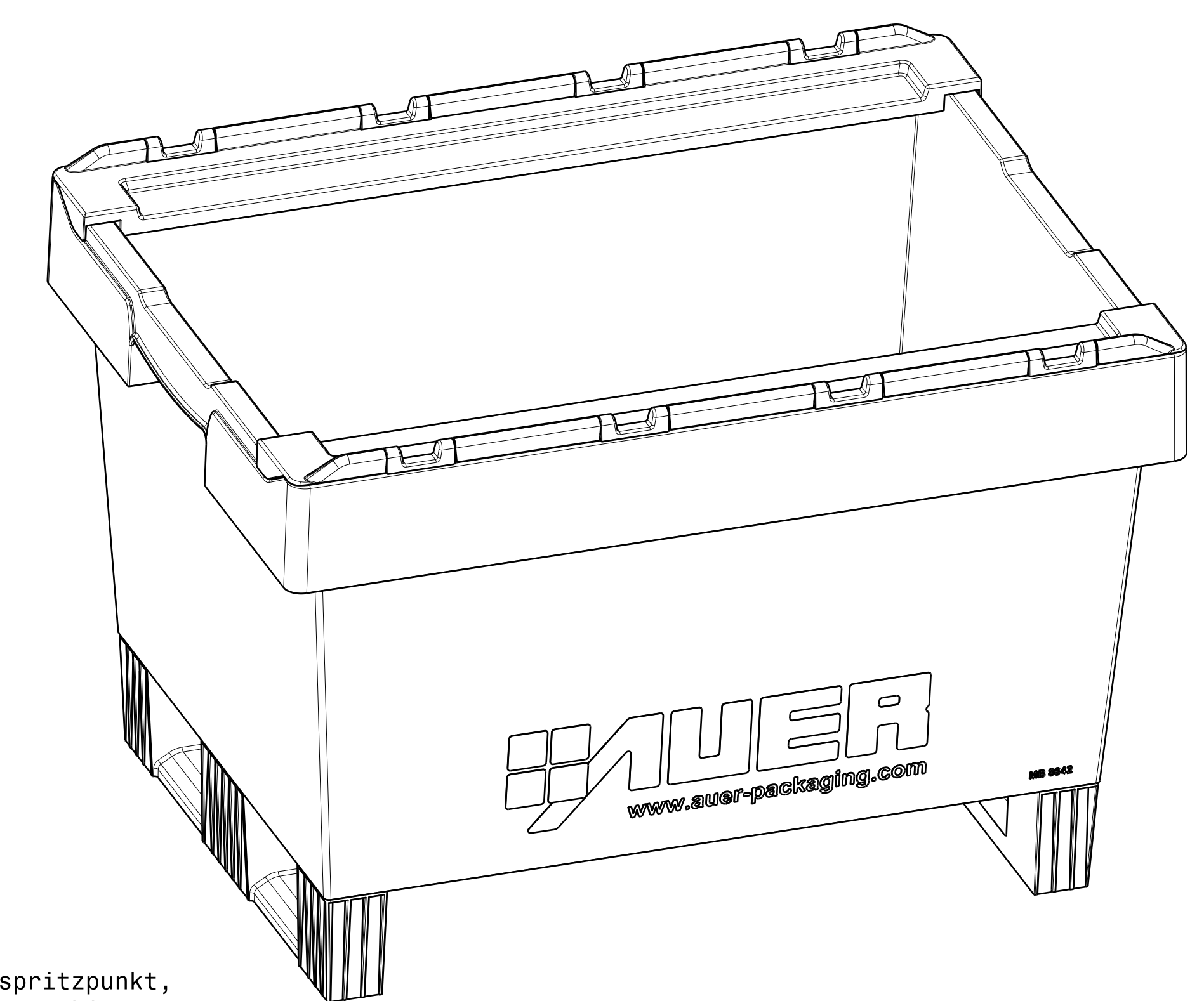
Isometrische Ansicht Maßstab: 1:4
