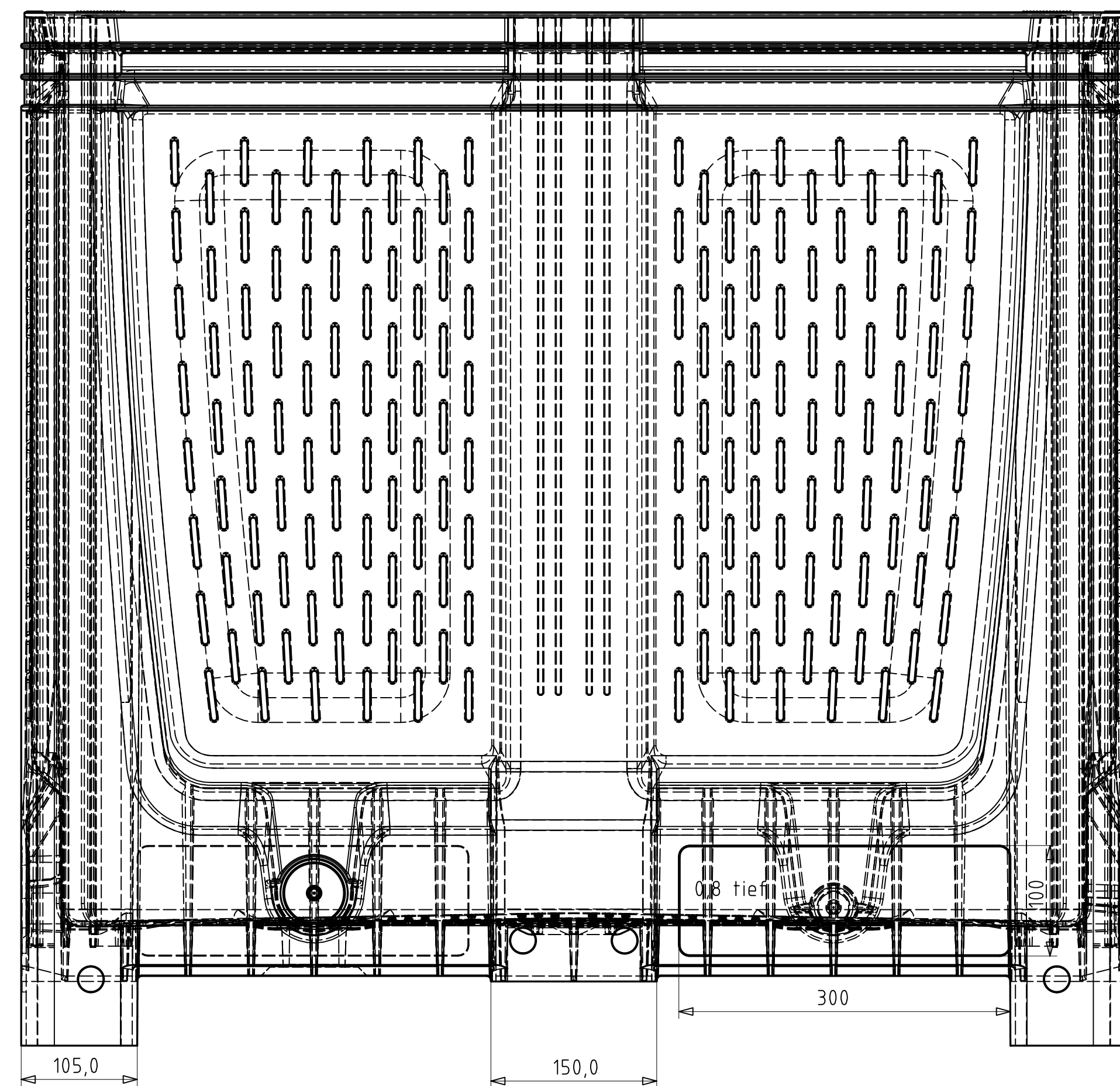
Schnitt B-B
