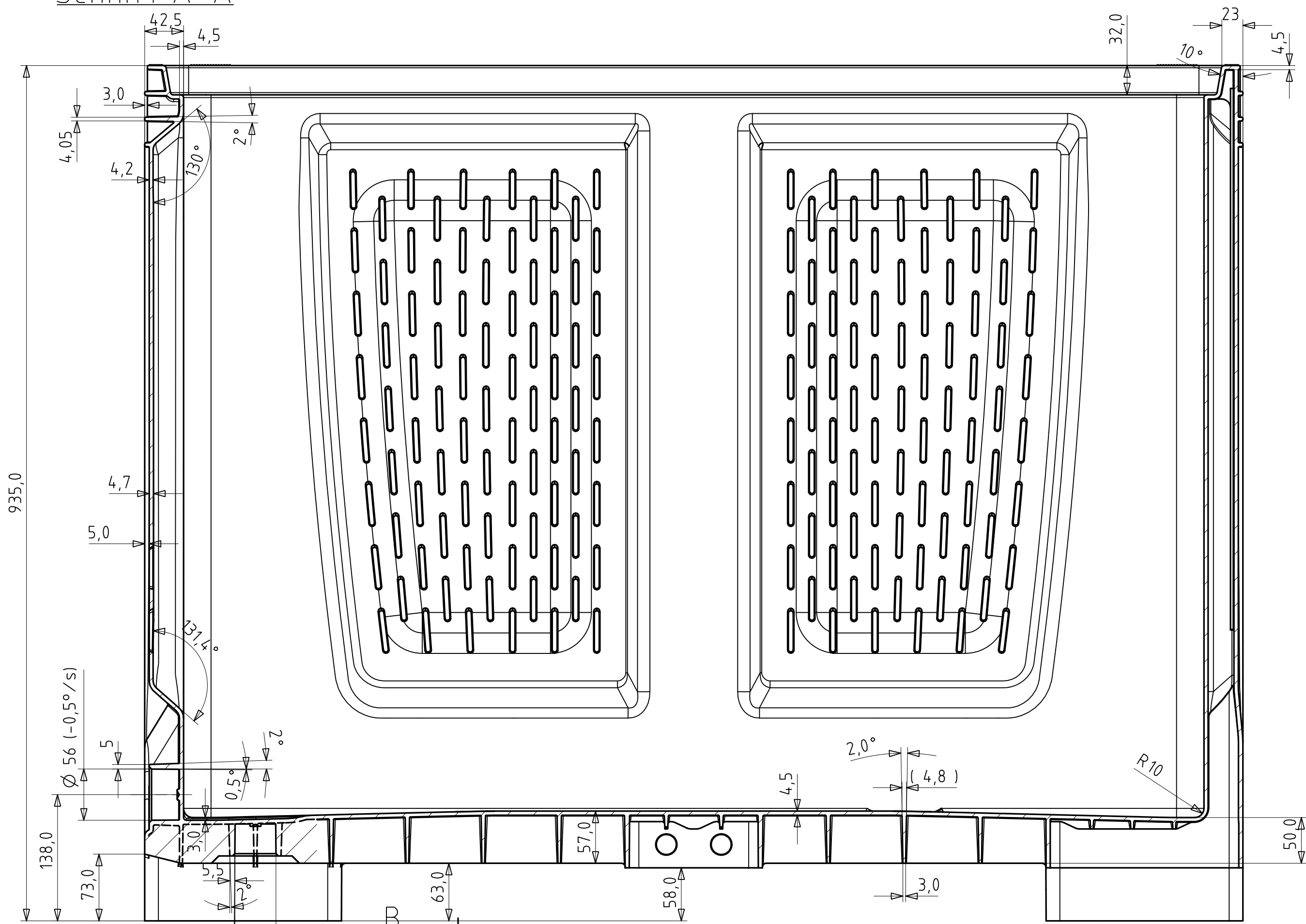
Schnitt A-A
