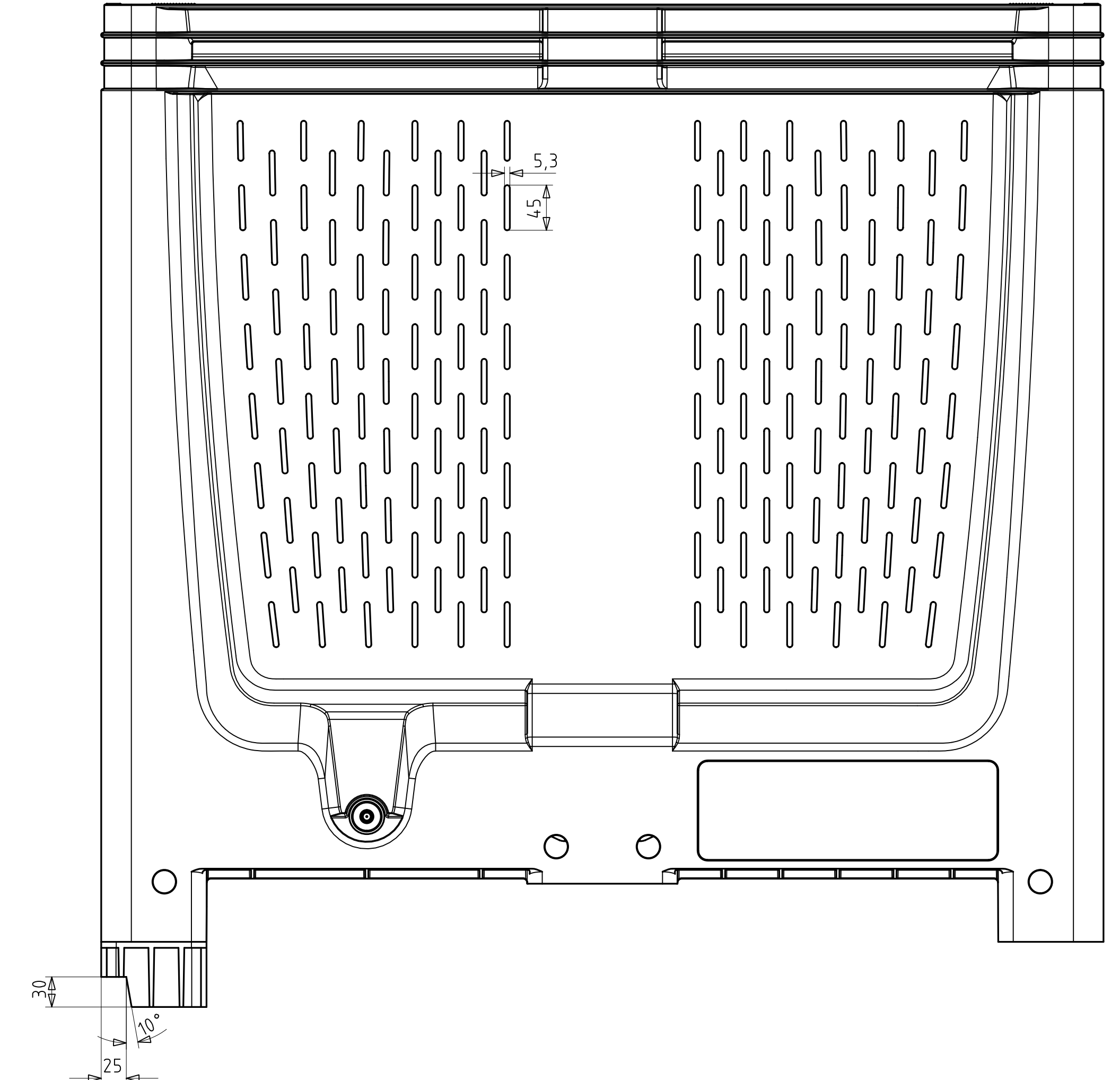
Schnitt D-D
