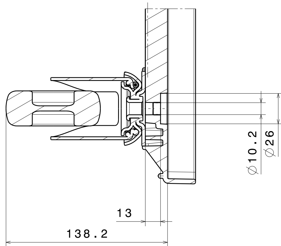
Schnittansicht A-A
